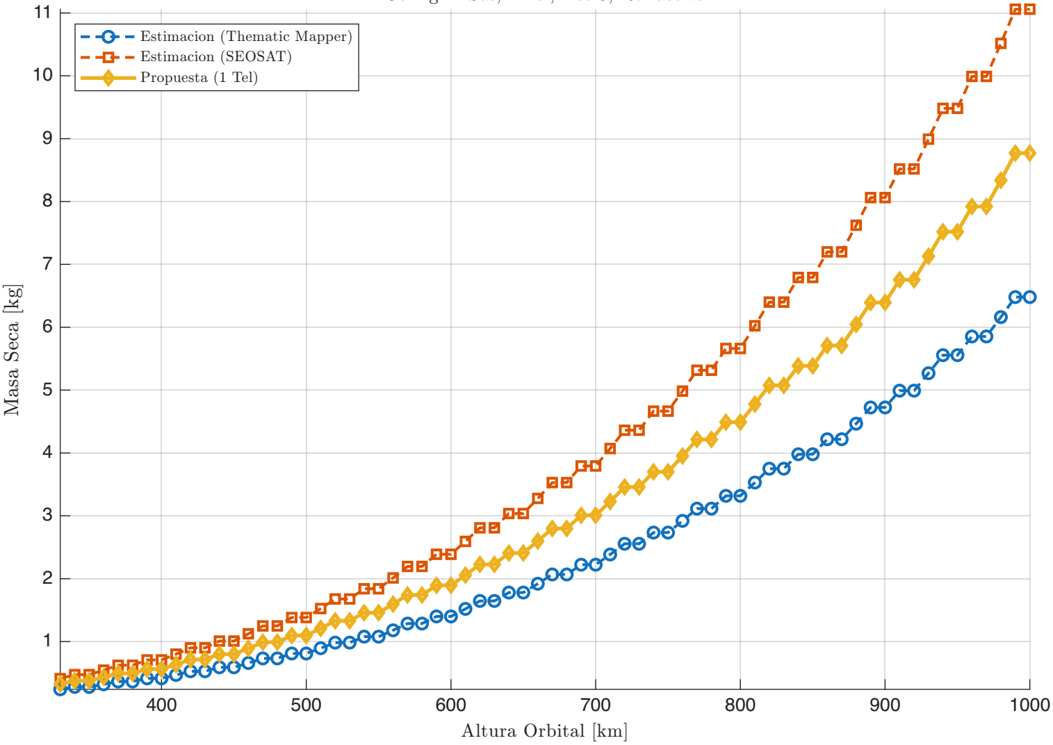
Comparativa de Masa Seca vs. Altura Config: 1 Sat, 1 Tel, Det 3, Refractivo
